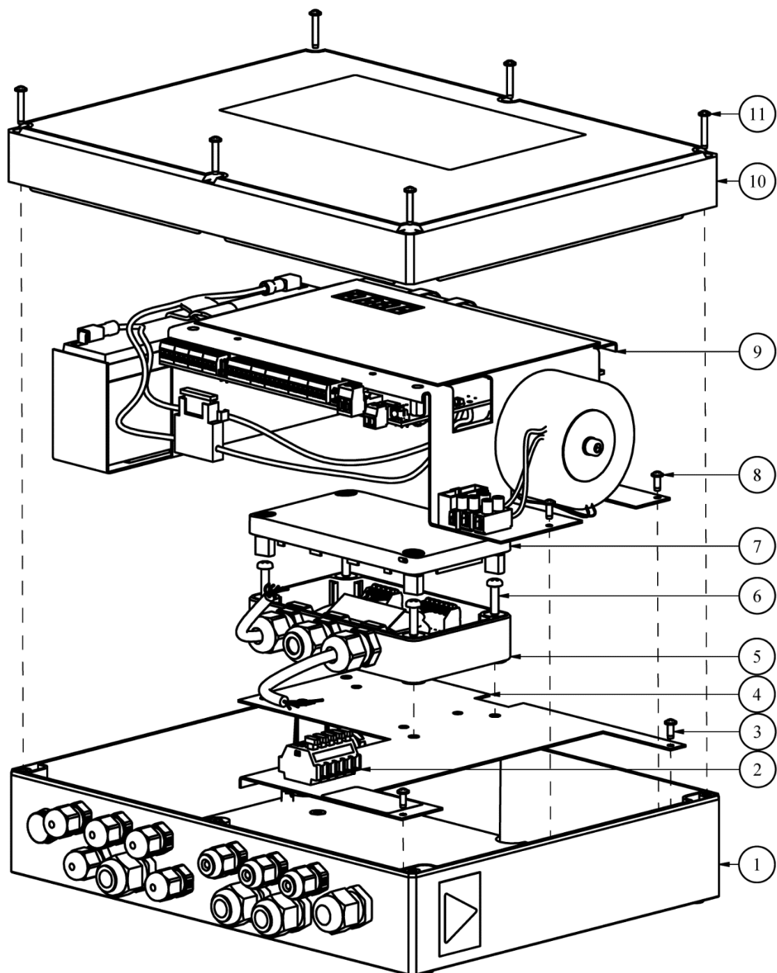
Rysunek 10.1/1 Schemat montażu AKC-6000 w centrali detekcji gazów CDG 6000-16
